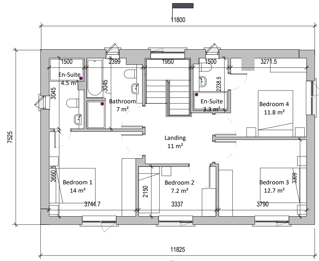
2 H07 Level 01 1 : 100
